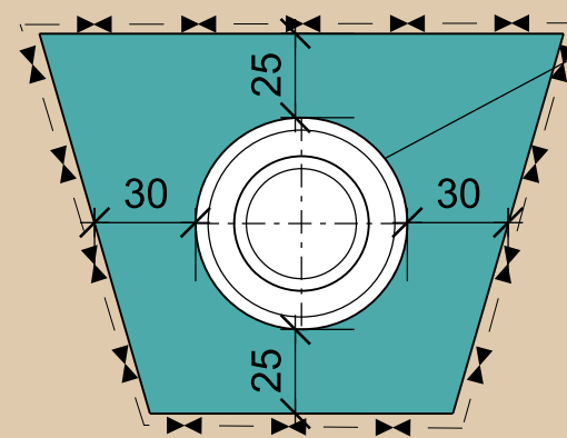
Sickerwasserableitung Sauger 1 - 4 Mantel-/Medienleitung, PE 100 RC, SDR 17/11, DA 630/400
