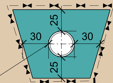
Schichtwasserausleitung Sauger 1 - 4 PP, DN 300, SN8, Vollrohr
